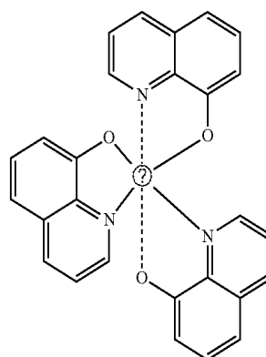
Alq 3
